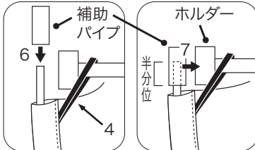
6. 補助パイプを湾曲した部材の端にパイプの長さの半分程度通して
